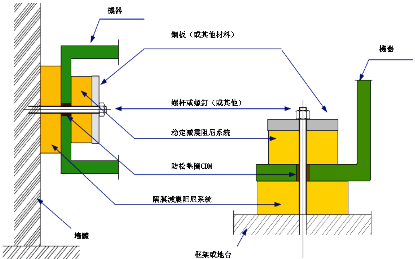
CDM-ISO-MACHINE-FIX的縱橫設計圖
